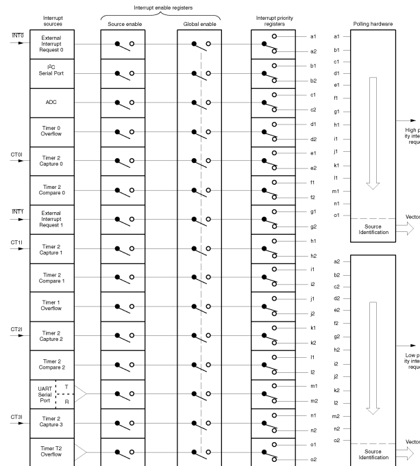
Abbildung 6.4: Darstellung der Interruptverarbeitung [1]
