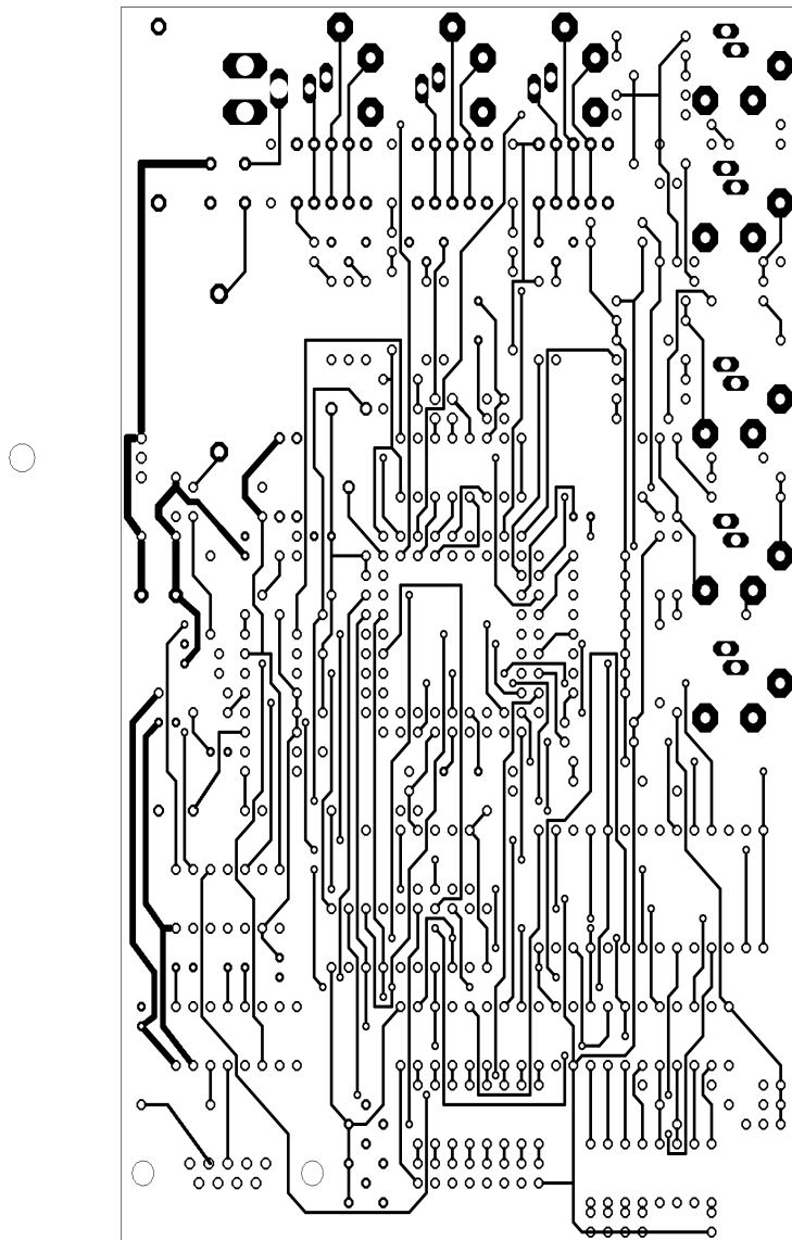
Abbildung 12.3: Lötseite der Endversion
