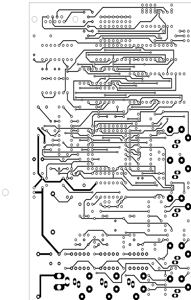
Abbildung 12.2: Bauteilseite der Endversion
