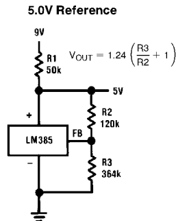
Abbildung 11.2: Beispielschaltung für die Dimensionierung der Referenzspannungsquelle [2]
