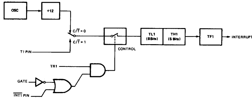
Abbildung 9.2: Darstellung zum Mode 1 der Timer 0 und 1 [9]
